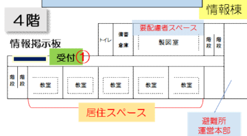
配置計画図 (例)
