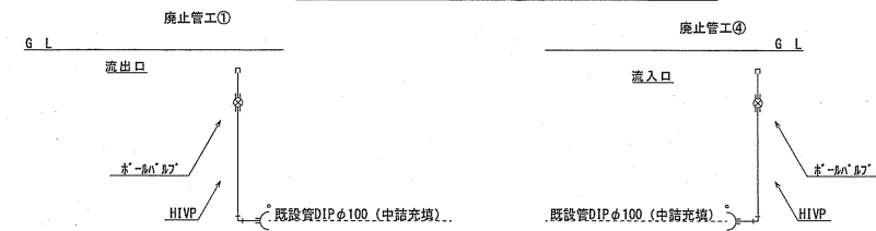
既設管廃止図 (中詰充填) S=1:Free
