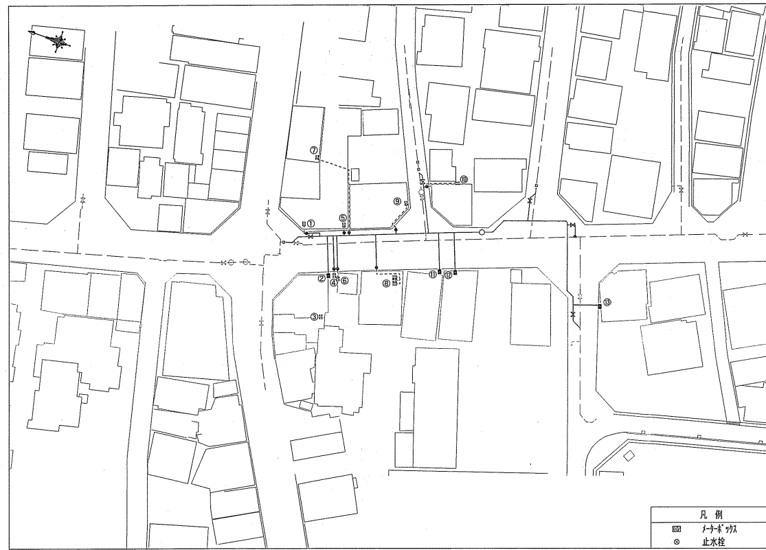
給水切替平面図 S=1:500
