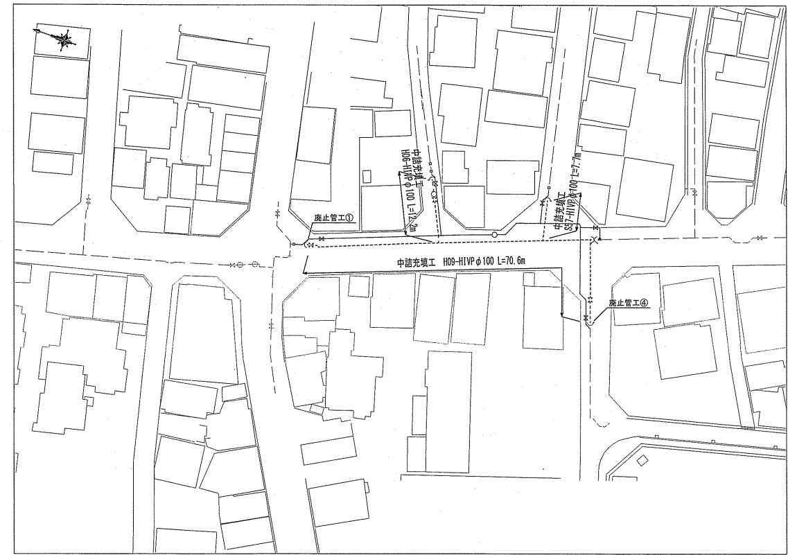
既設管廃止工平面図 S=1:500
