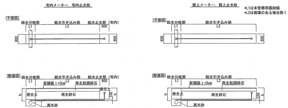
切替標準断面図 S=Free
