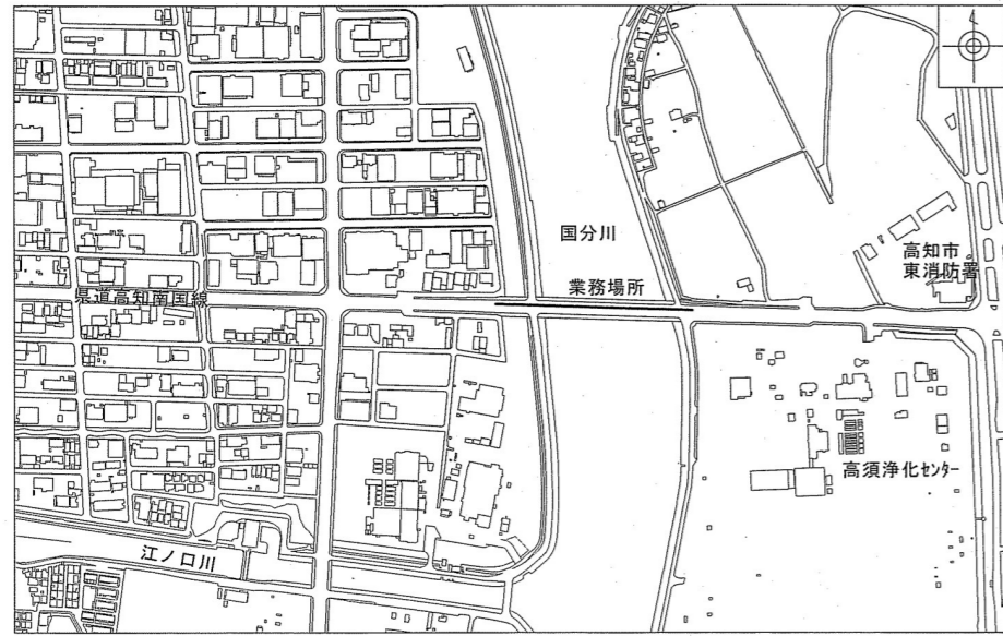
平面図 S=1:1000
