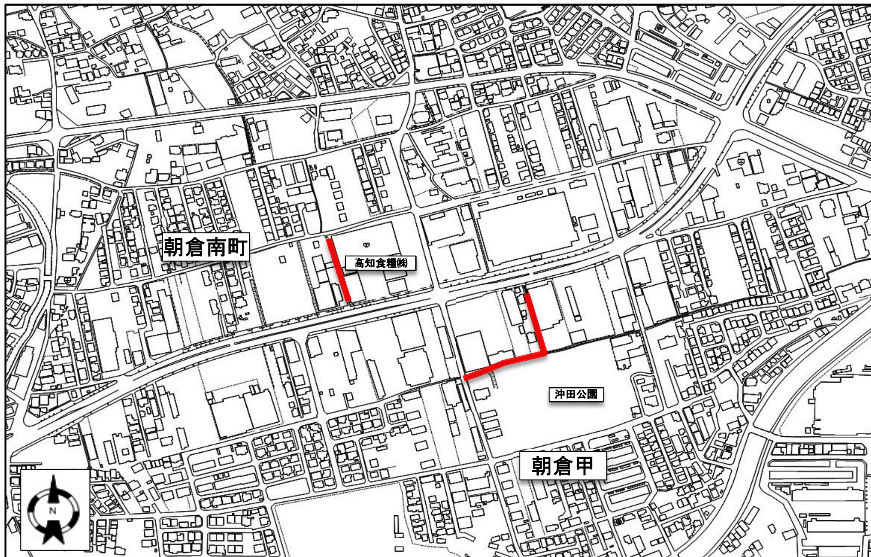
位置図 令和6年度 朝倉分区污水管渠築造工事(R6-7)
