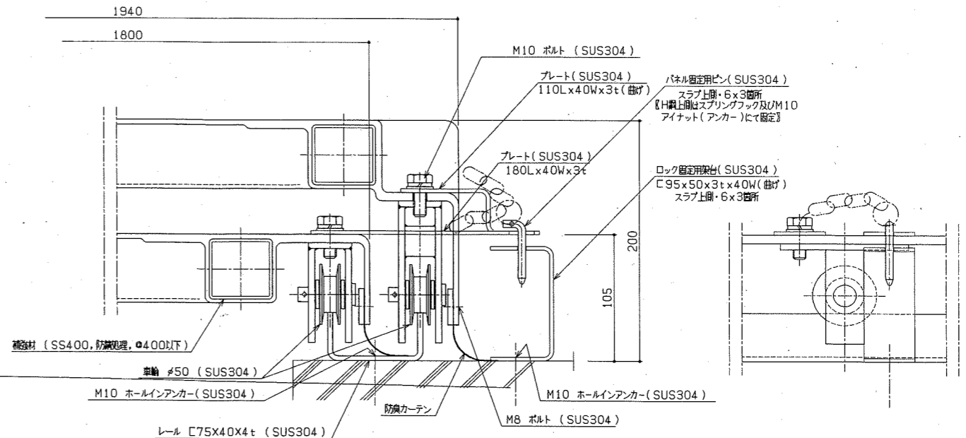
車輪取付詳細
