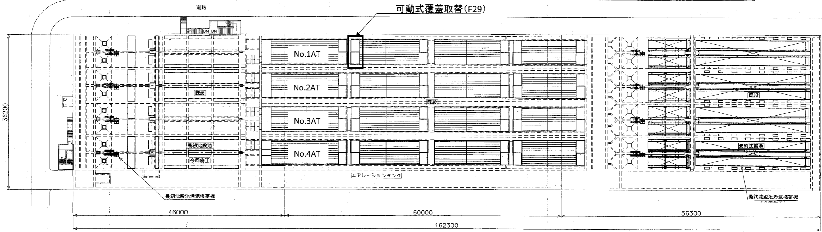
全体配置平面図
