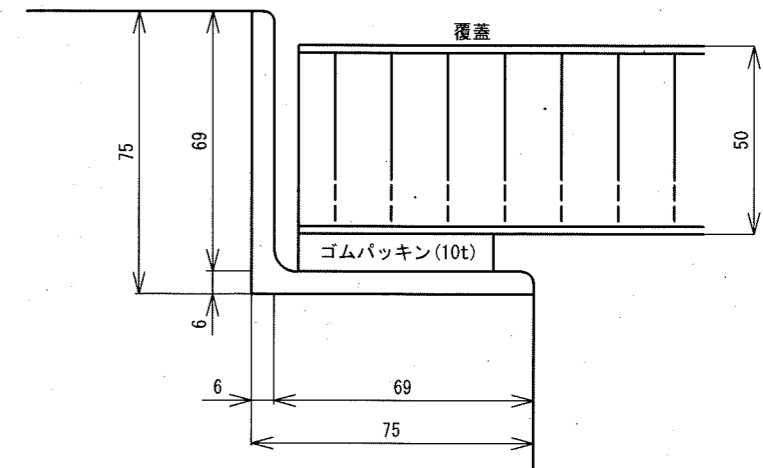
既設受枠詳細
