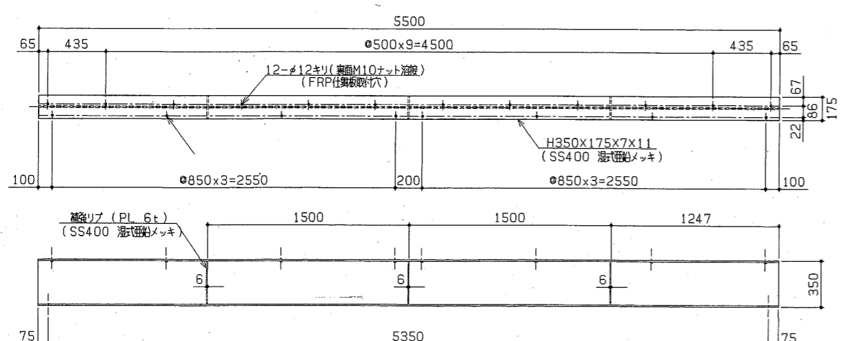
鋼材詳細
