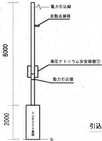
引込柱①詳細図 NS
