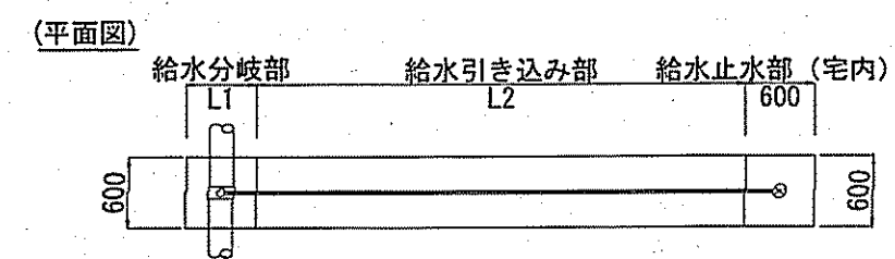
宅内メーター、宅内止水栓
