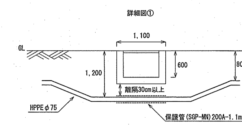
詳細図 S=1:Free
