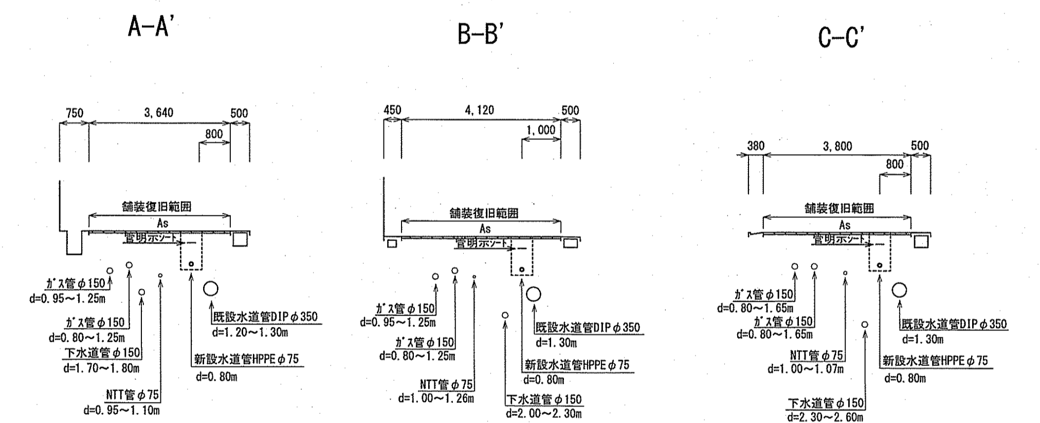
横断面図 S=1:100
