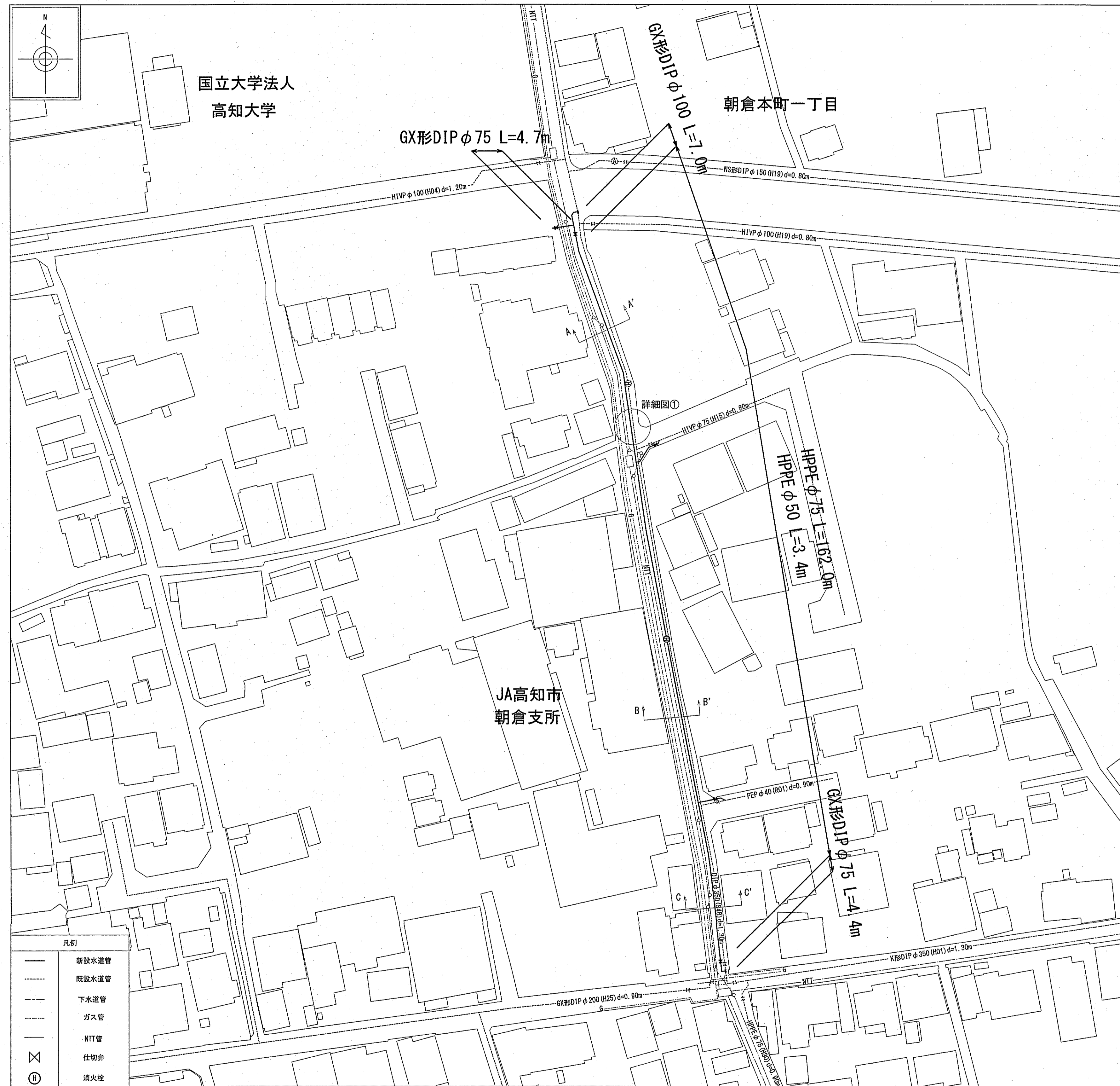
平面図 S=1:500
