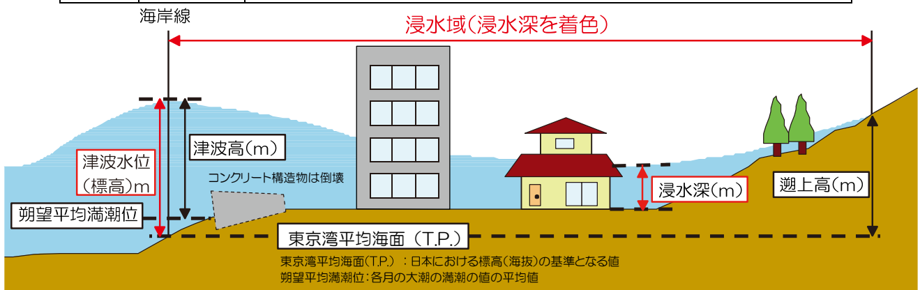
図 3-1 津波高及び津波浸水深のイメージ
