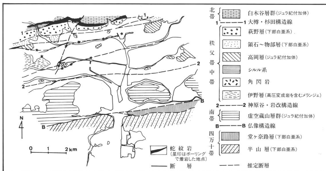
図4-1 高知平野周辺部の基盤地質図
