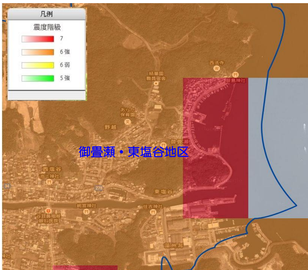
図9 御豊瀬・東塩谷地区における震度分布図
