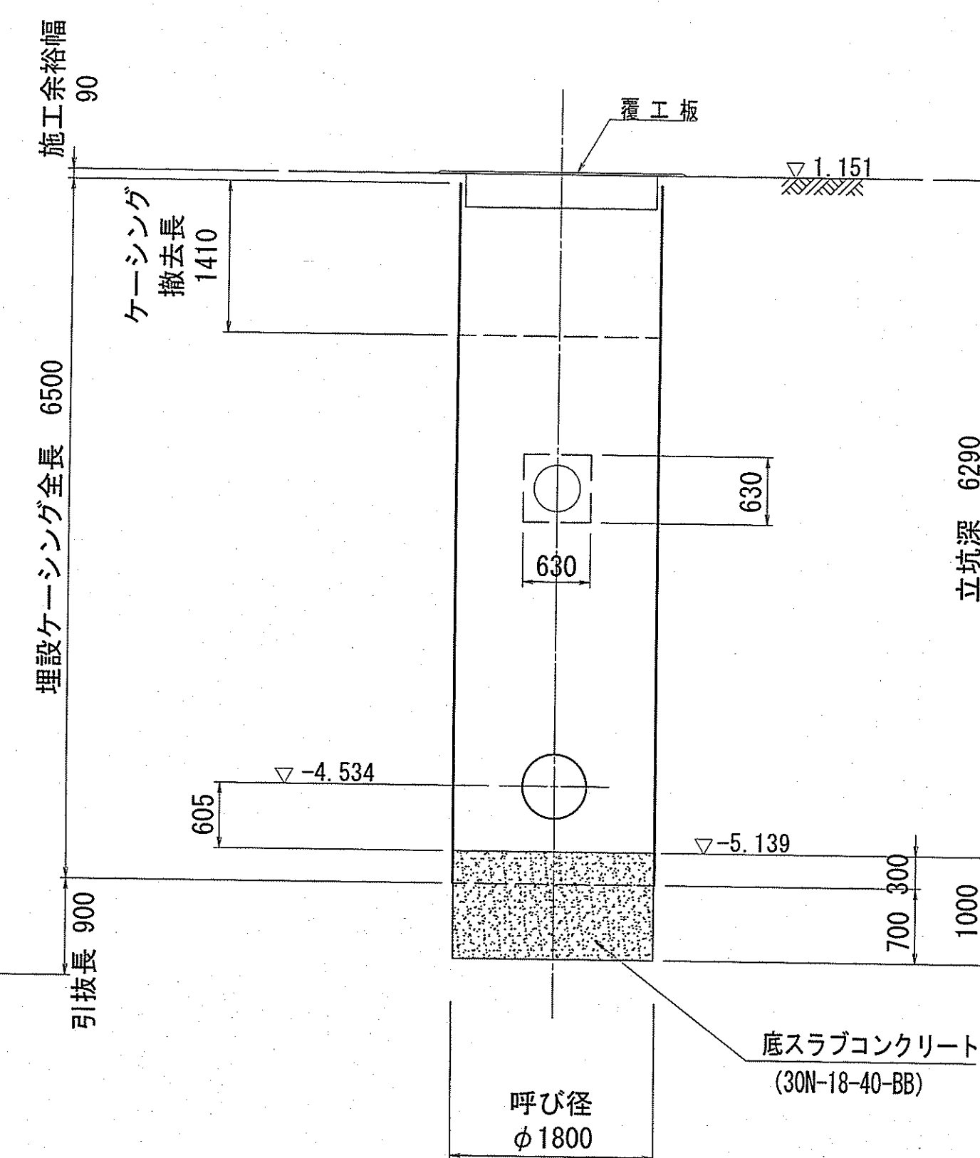
A-A断面図
