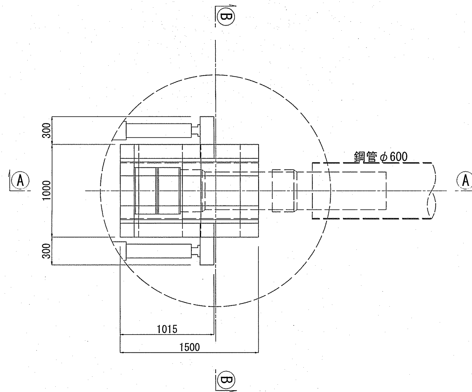
管挿入時 (1.0m管挿入)
