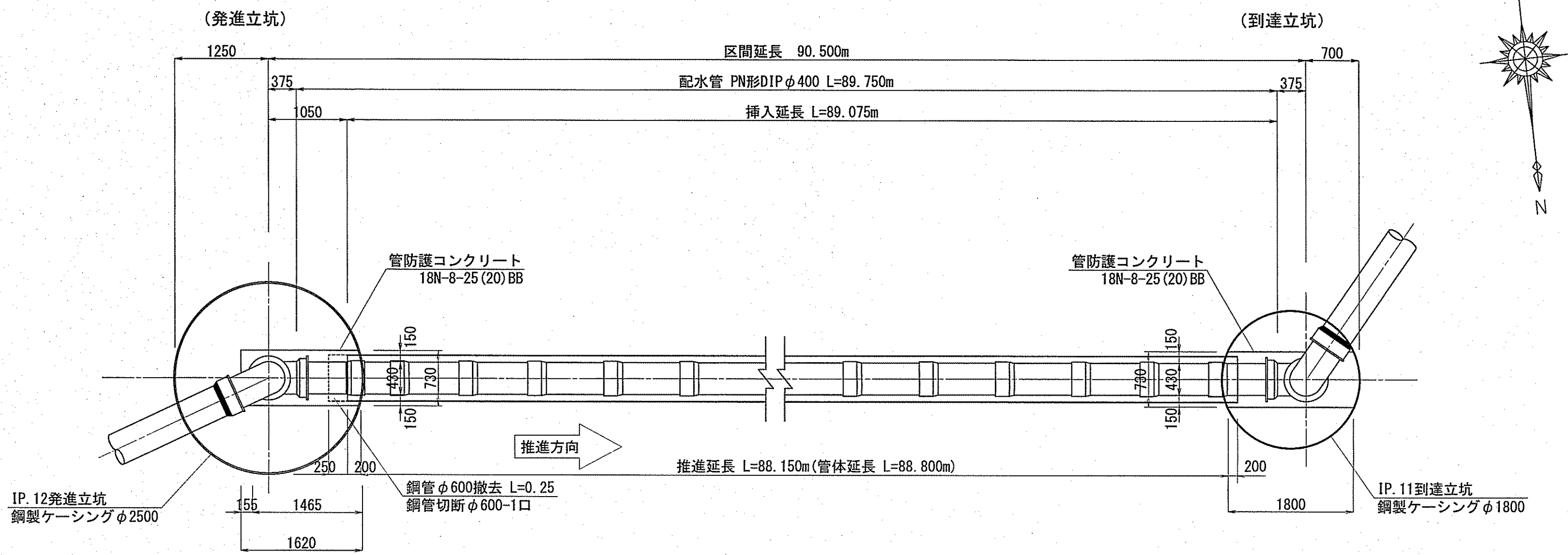
平面図
