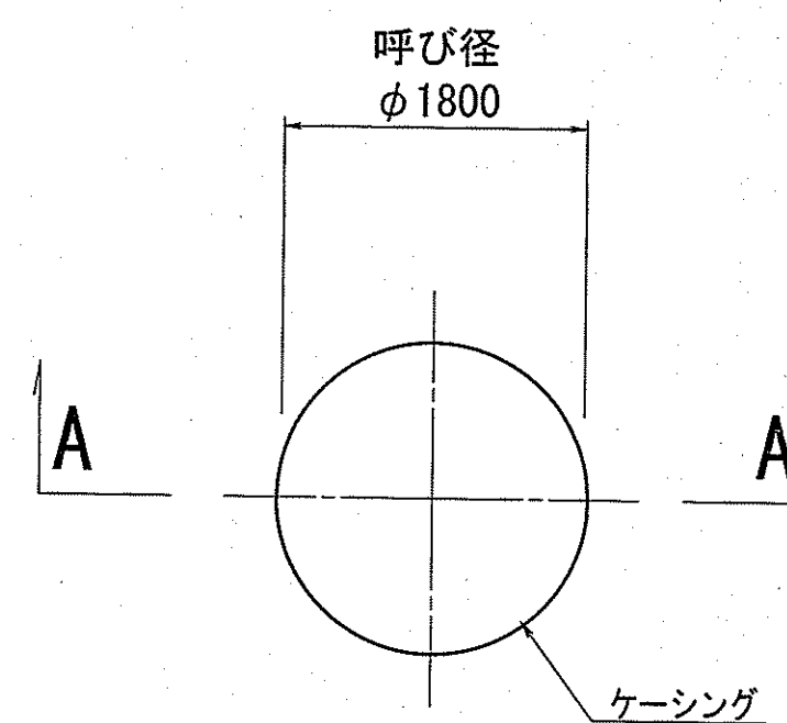
平面图
