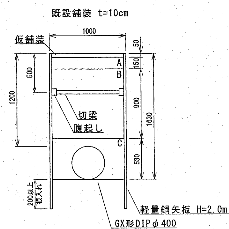
GX形φ400布設 (d=1.20m) L=43.630m
