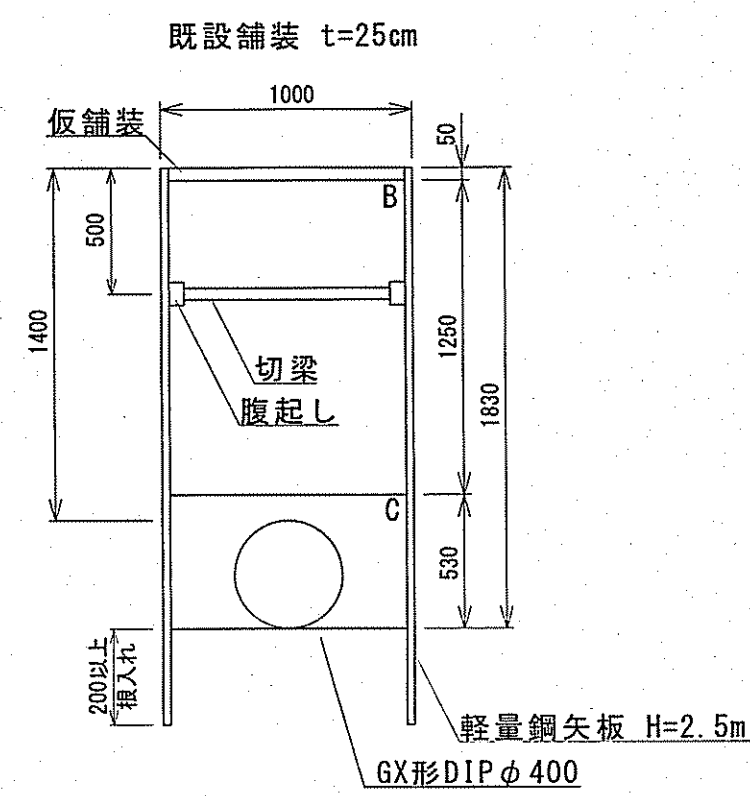
GX形φ400布設 (d=1.40m) L=12.750m(改良部)
