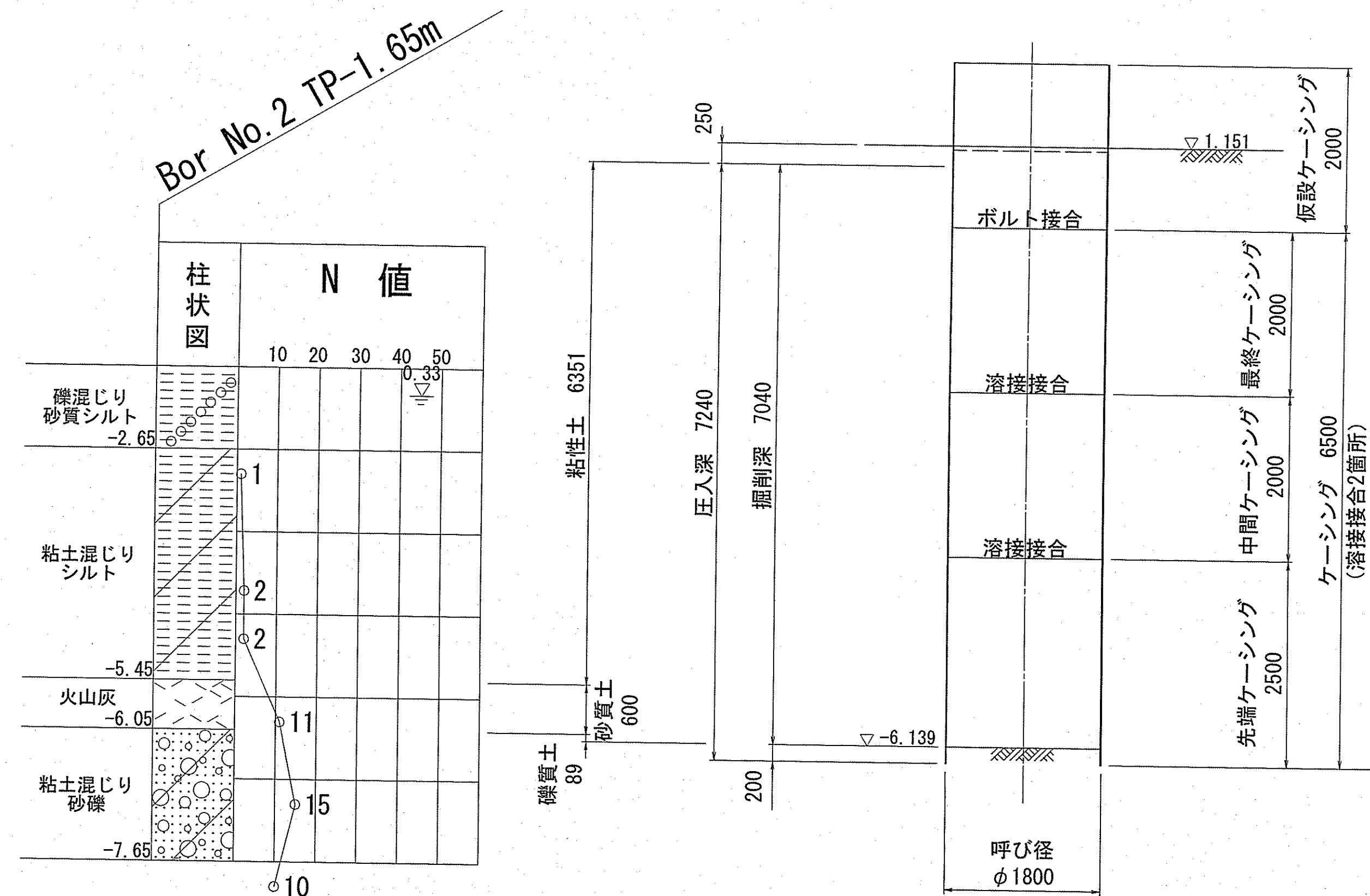
断面図
