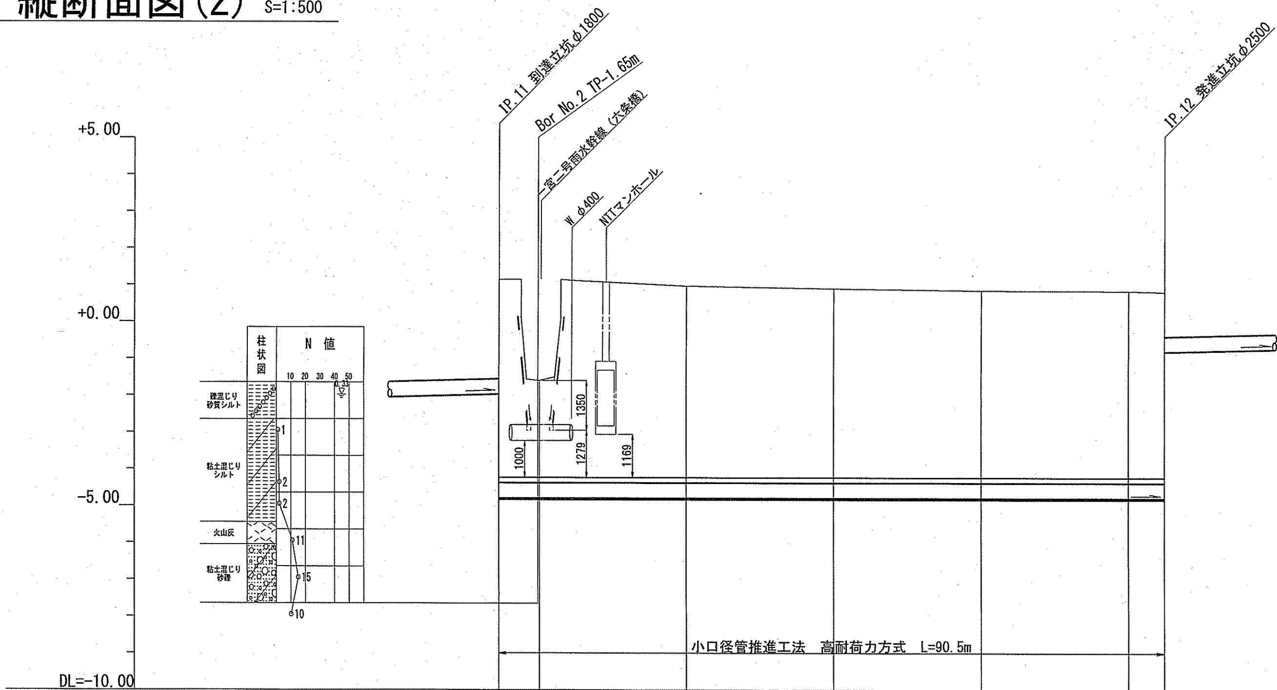
縦断面図(2) V=1:100 S=1:500
