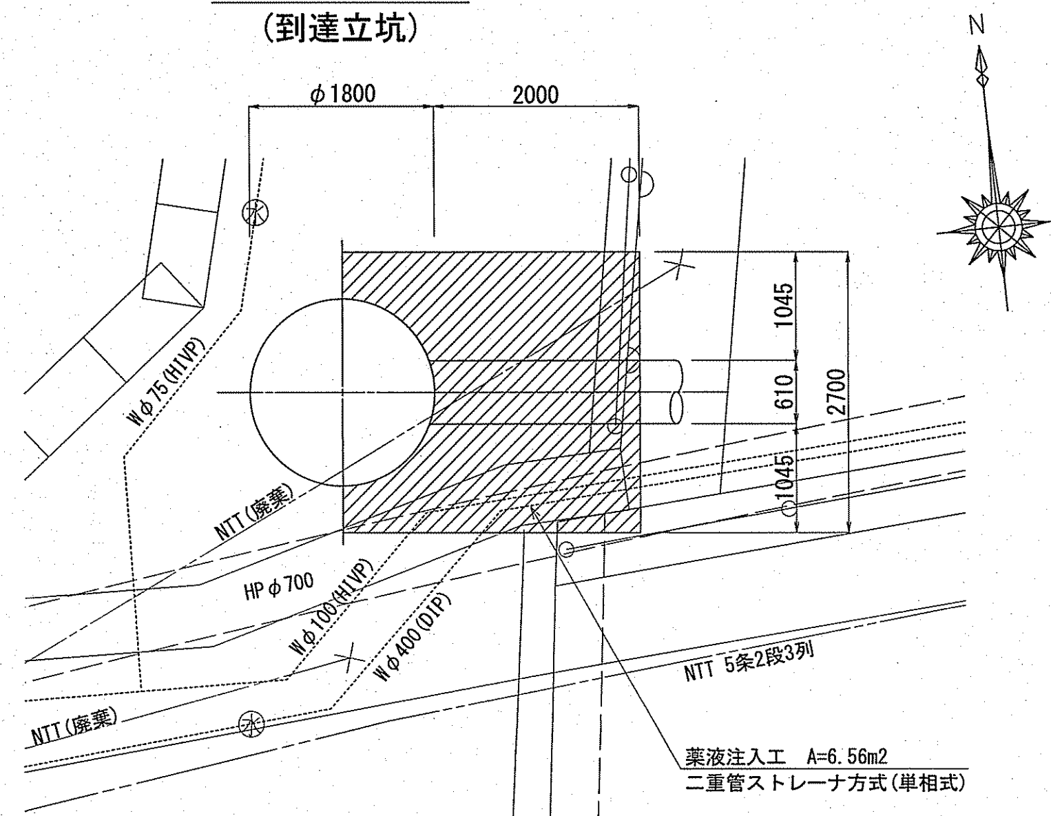
断面図 (到達立坑)
