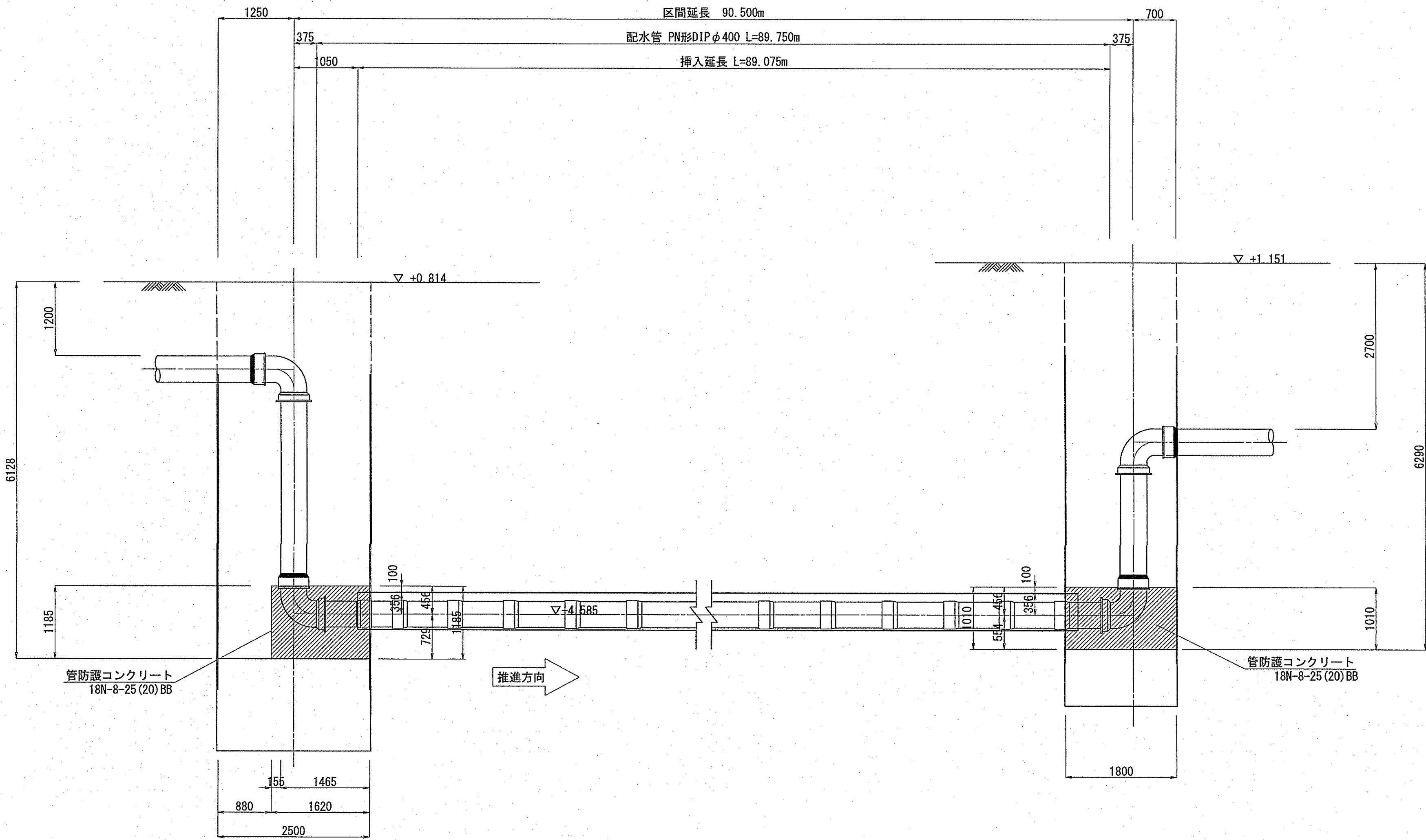
断面図
