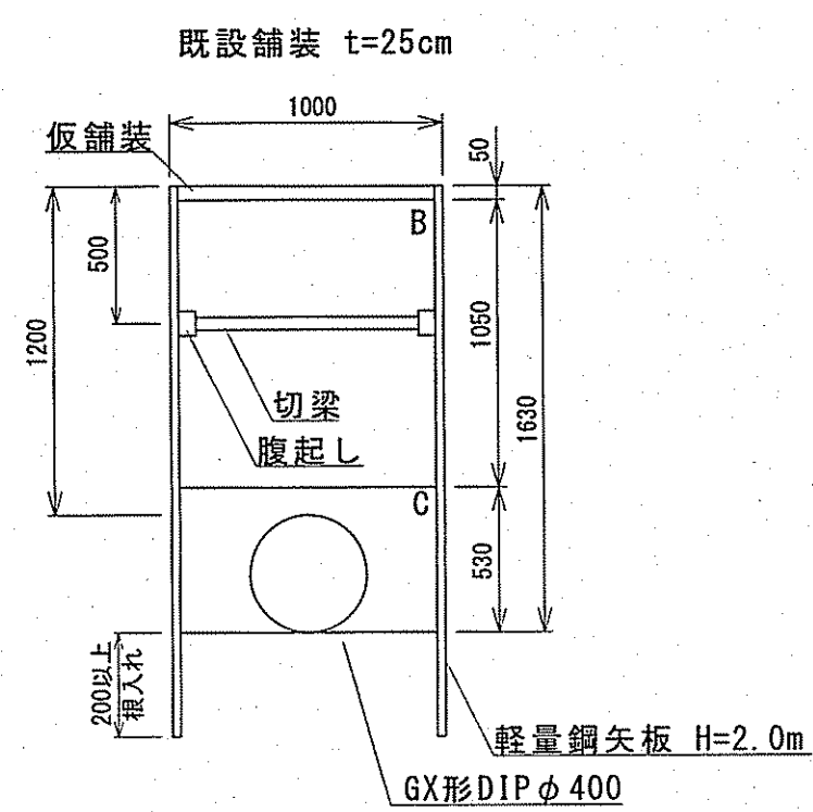
GX形φ400布設 (d=1.20m) L=57.155m(改良部) (15.210m+41.945m)
