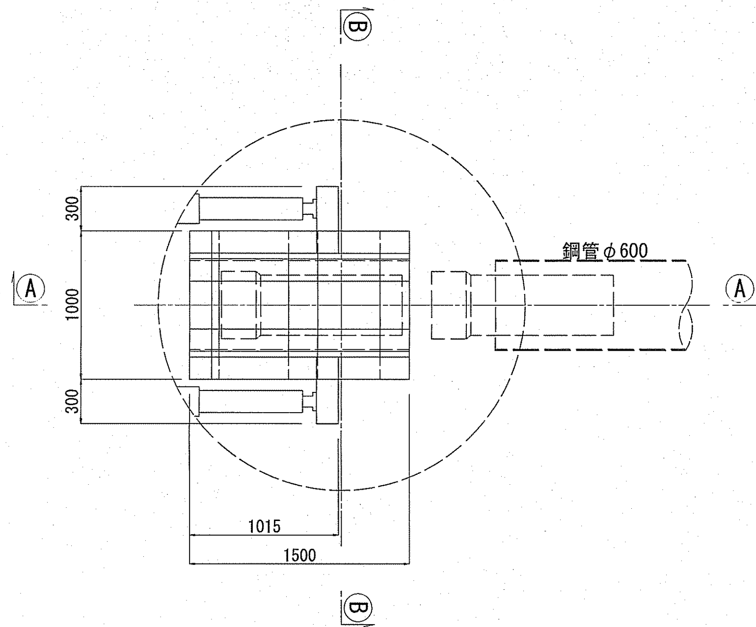
管据付時 (1.0m管挿入)
