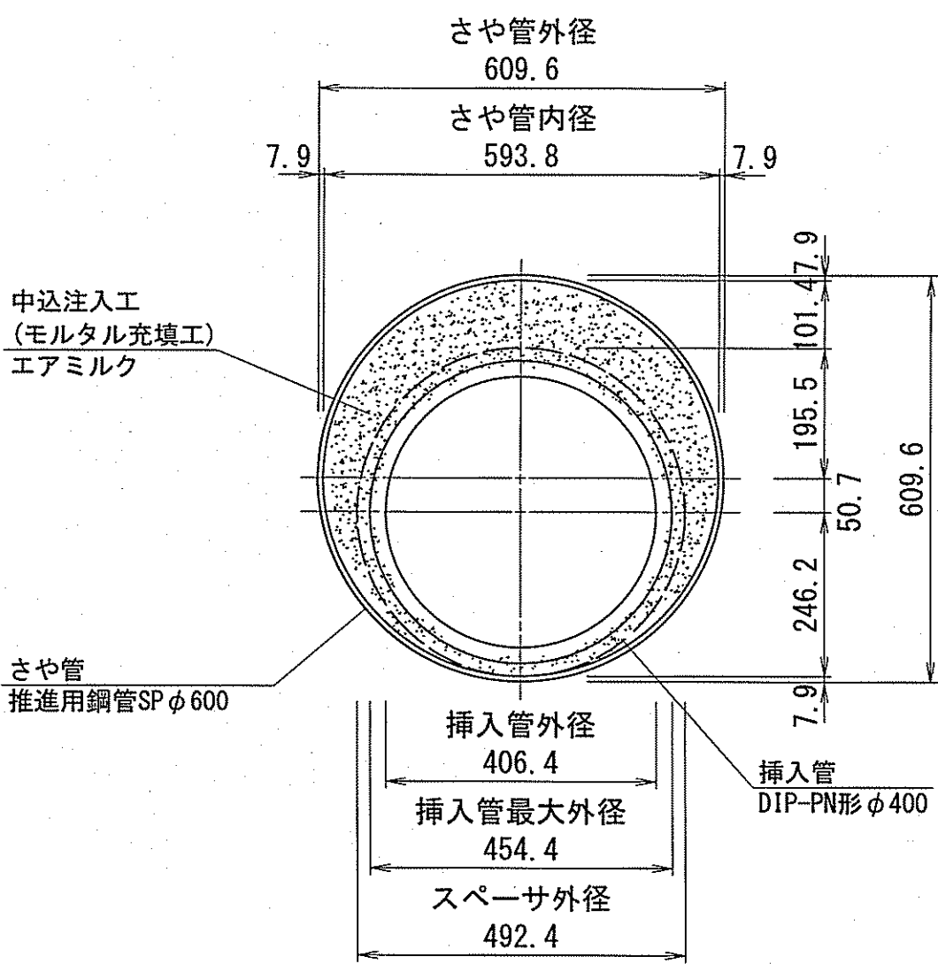
推進管内配管断面図 S=1:10 (参考図)
