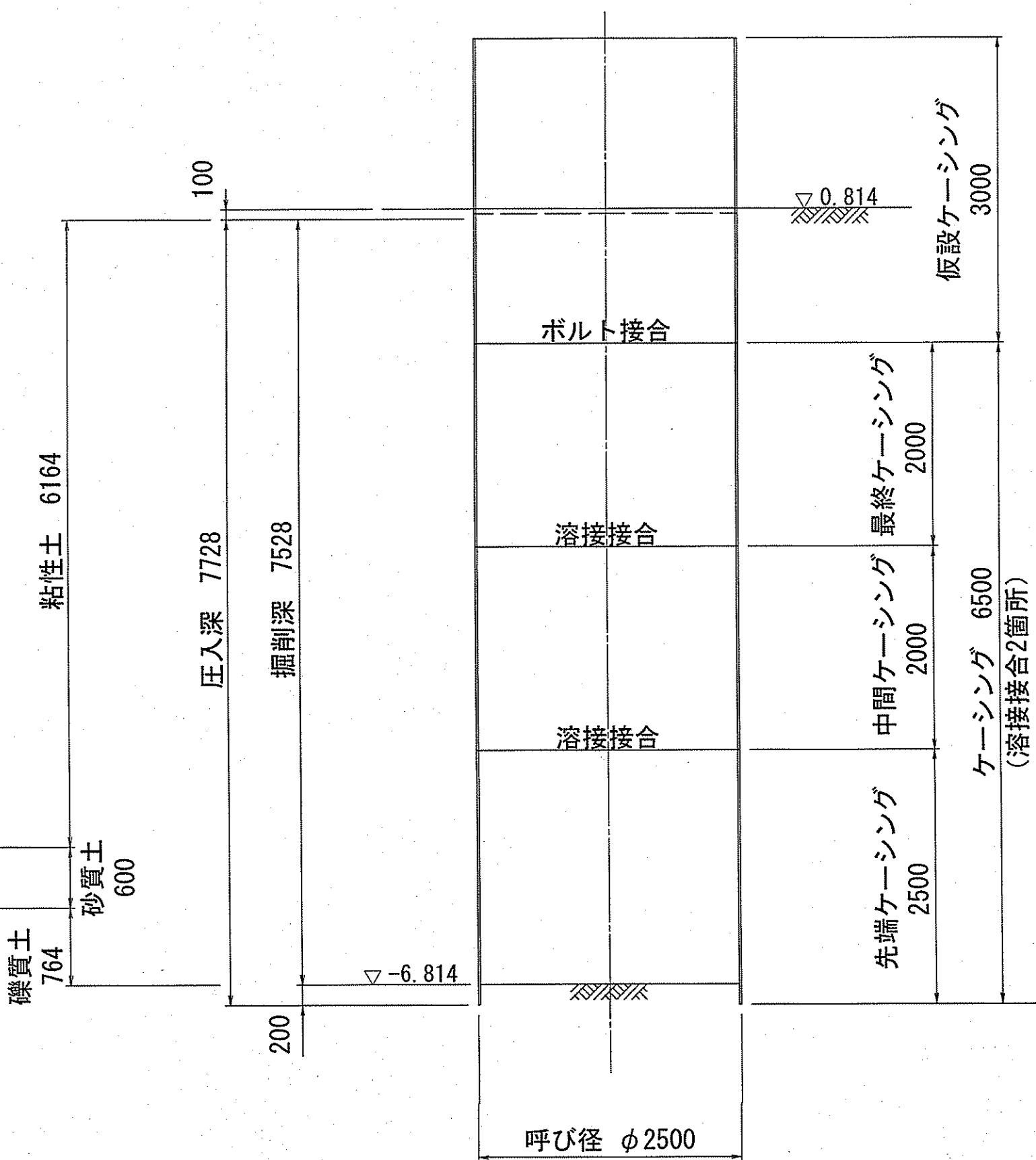
断面図
