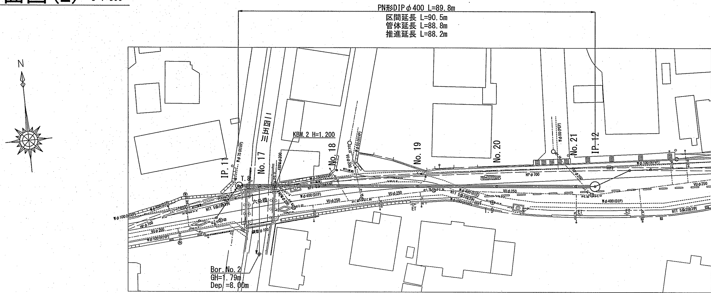
平面図(2) S=1:500
