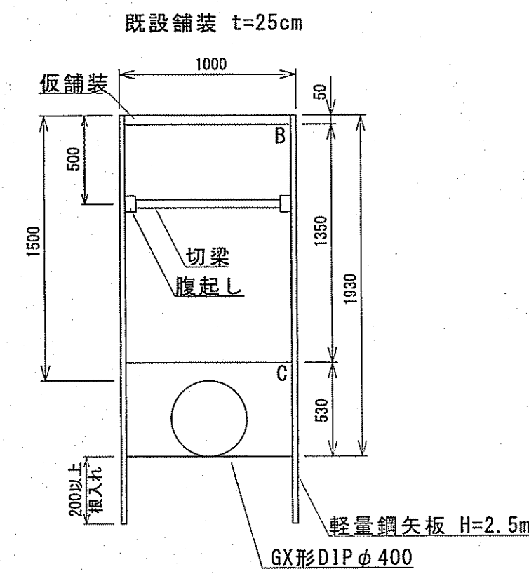
GX形φ400布設 (d=1.50m) L=3.095m(改良部)
