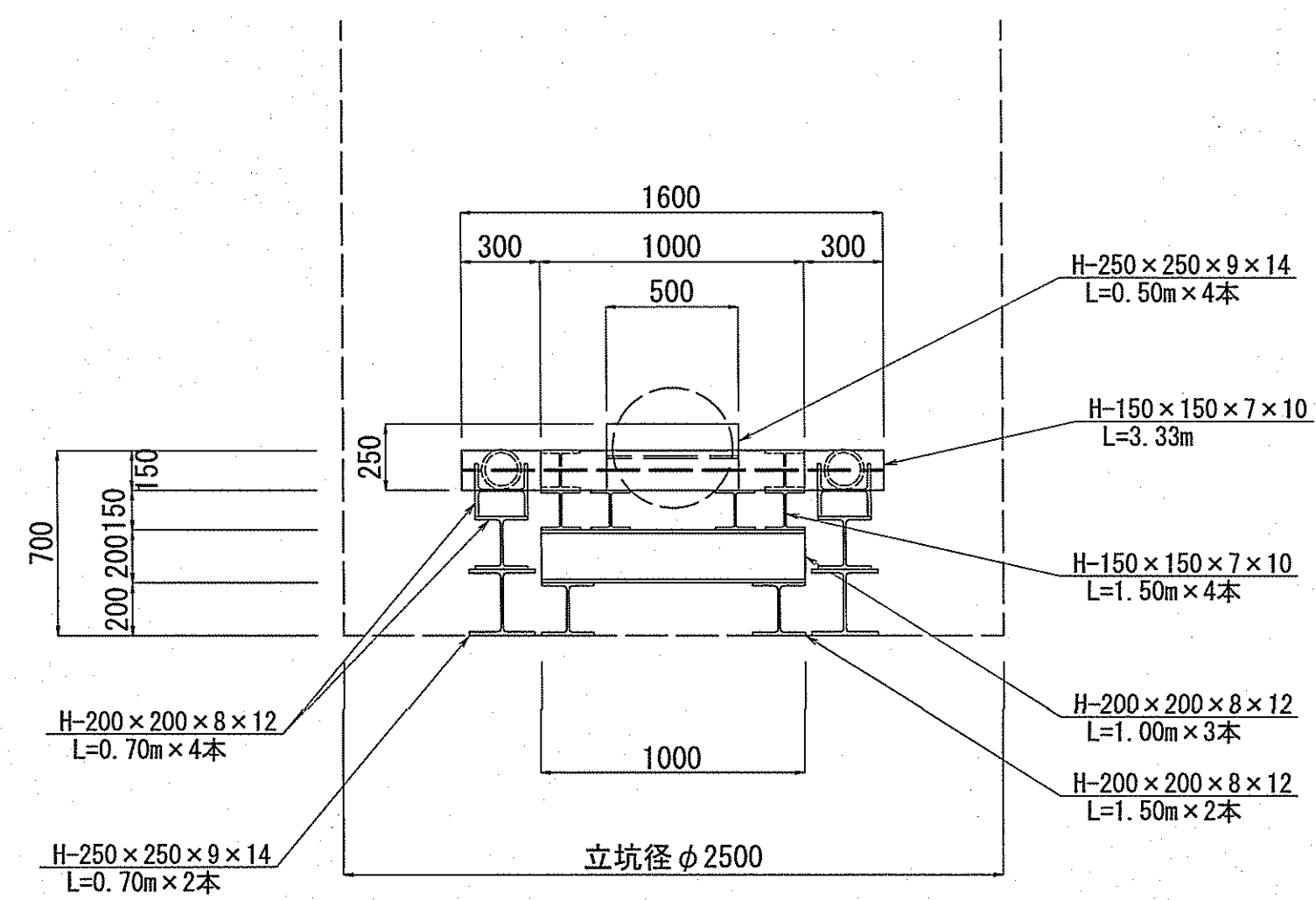
②-② 断面図
