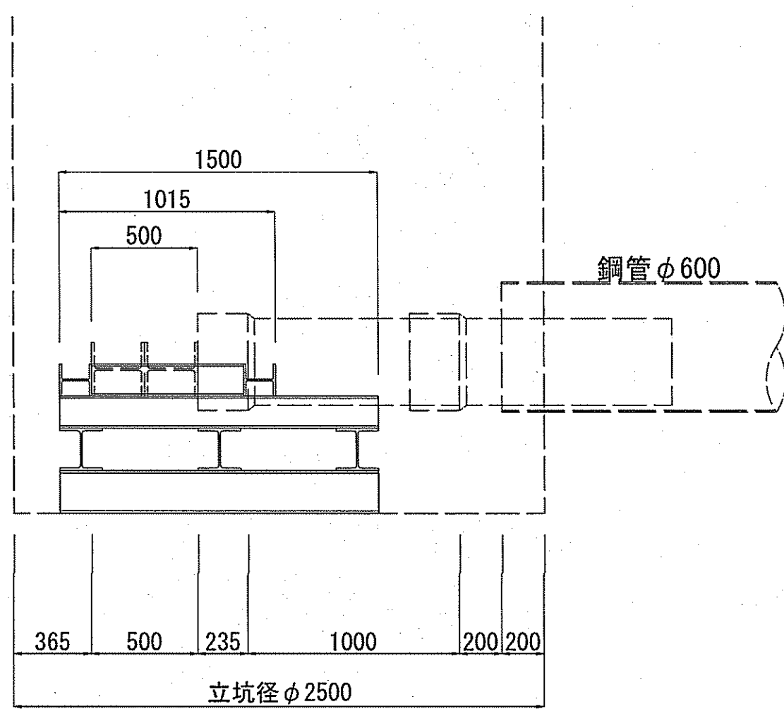
①-① 断面図
